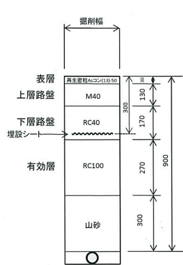
仮復旧図
