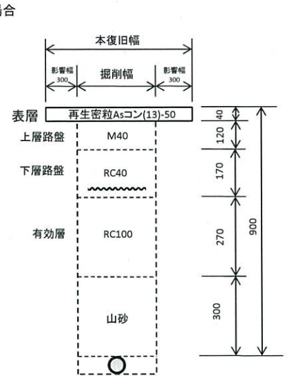
本復旧図
