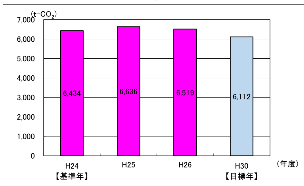
【市役所からの排出量 (t-CO 2 )】
