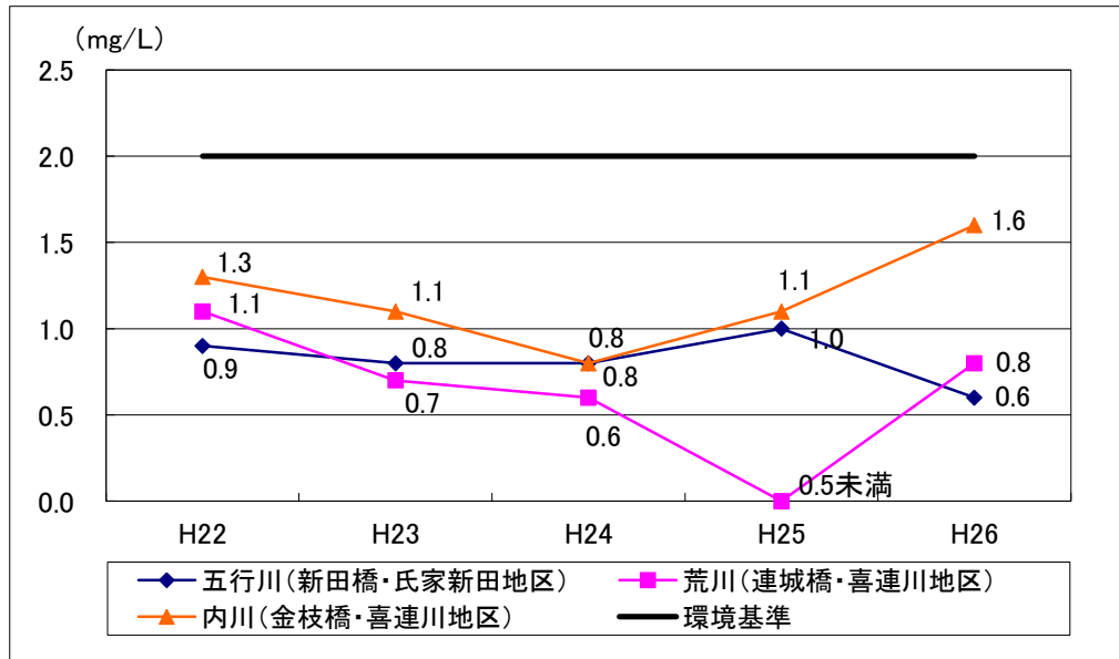
【水質調査結果 (BOD*) の推移】
