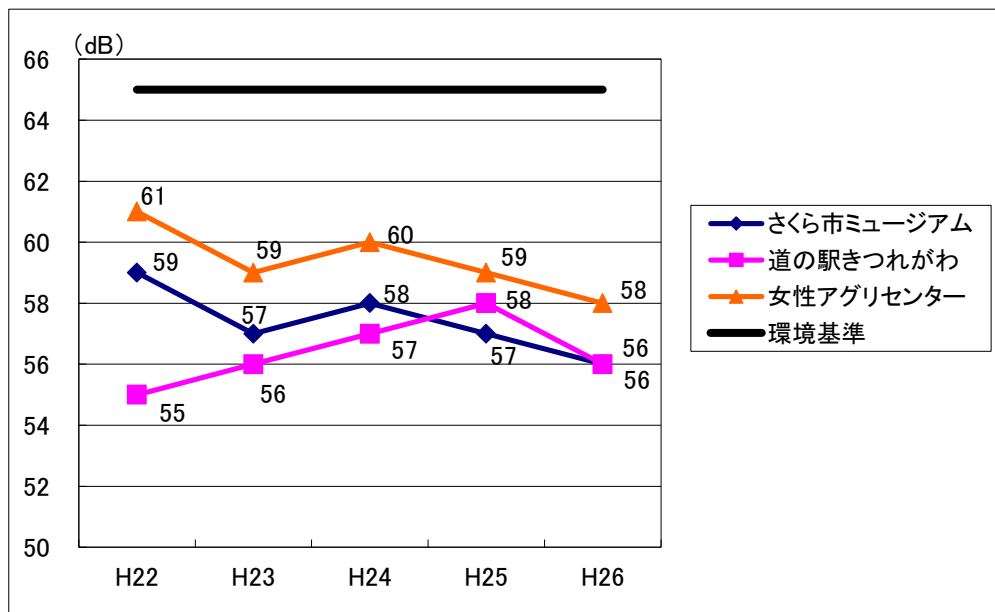
【騒音調査結果（夜間）の推移】
