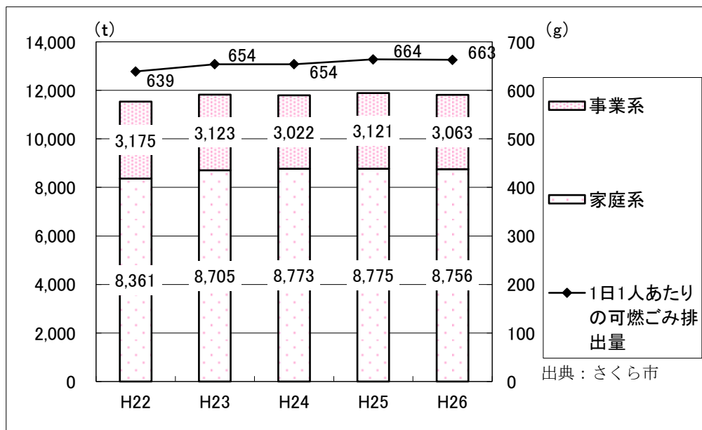
【家庭系ごみ及び事業系ごみの推移と1日1人あたりの可燃ごみ排出量の推移】
